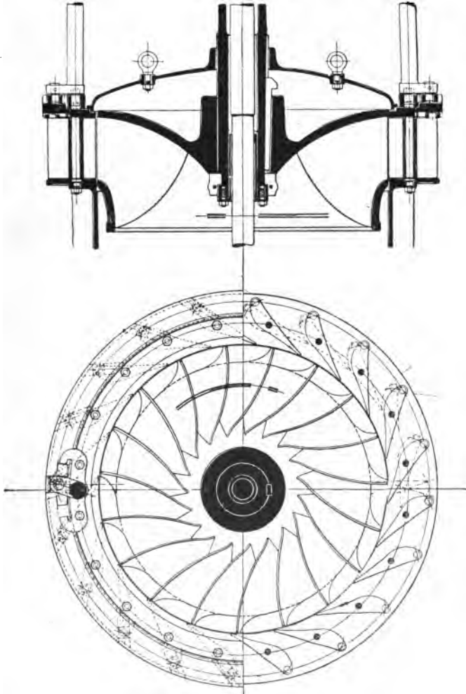
Fig. 46 und 47. Francis-Turbine.
